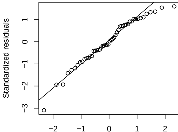
Normal Q-Q
